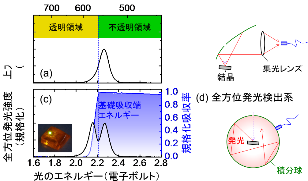
図 (a) 結晶の上方に放射された発光のスペクトル、(b) 標準的な発光スペクトル検出系、(c) 結晶の全方位発光スペクトル、(d) 全方位発光スペクトル検出系。
