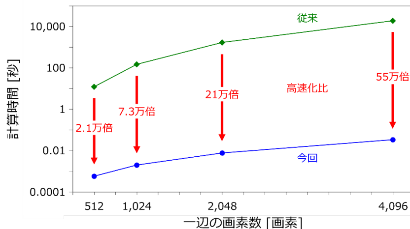
図1 計算時間の計測結果。いずれも10回計測した際の平均値を表す。グラフの横軸は光の情報を画像として表現した場合の一辺あたりの画素数、縦軸は計算時間。緑のひし形の点が従来の計算アルゴリズム、青の丸の点が開発した計算アルゴリズムによる計算時間の測定結果を表す。赤の矢印上に書かれている数値は、従来の計算アルゴリズムに対して開発した計算アルゴリズムが計算時間を何倍高速化できているかを表す。
